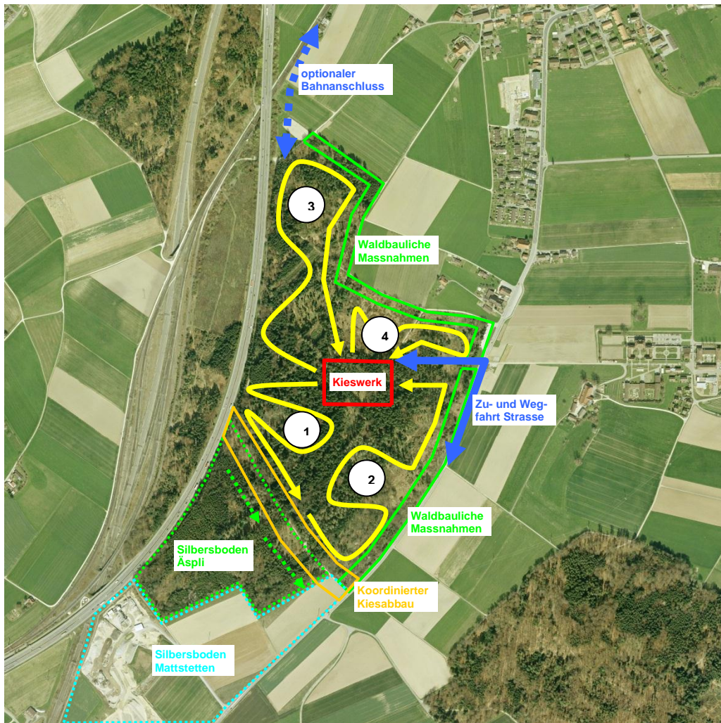
Abbildung 1: Abbauetappen, Abbaumethodik
